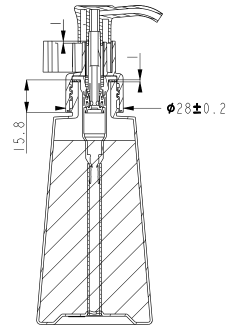
截面 B-B
