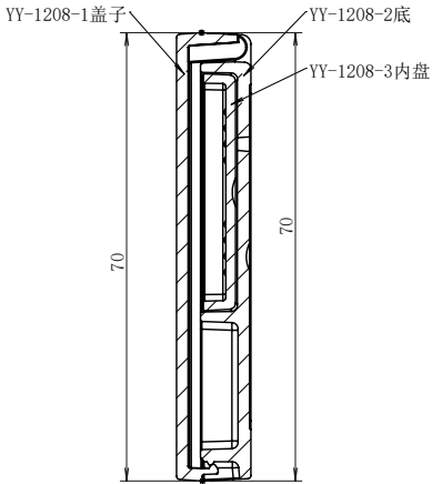
剖面 A-A
